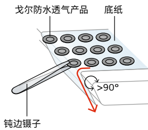
图2b: 弯折底纸
