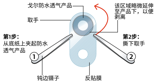
图9：取下取手（取手背面带有反贴膜）
