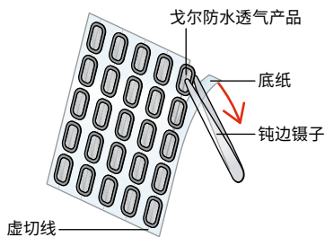
图3: 撕开底纸的虚切线
