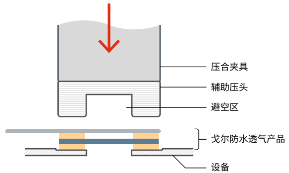
图6：带凹槽的辅助压头
