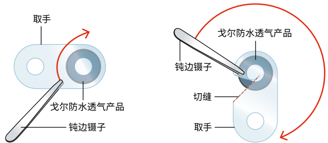
图7：取下无切缝取手
