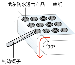
图2a: 弯折底纸
